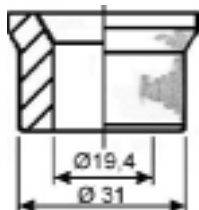
Reduzierhülse 2/5 44081 198 503 reducing sleeve 2/5 réducteur 2/5
